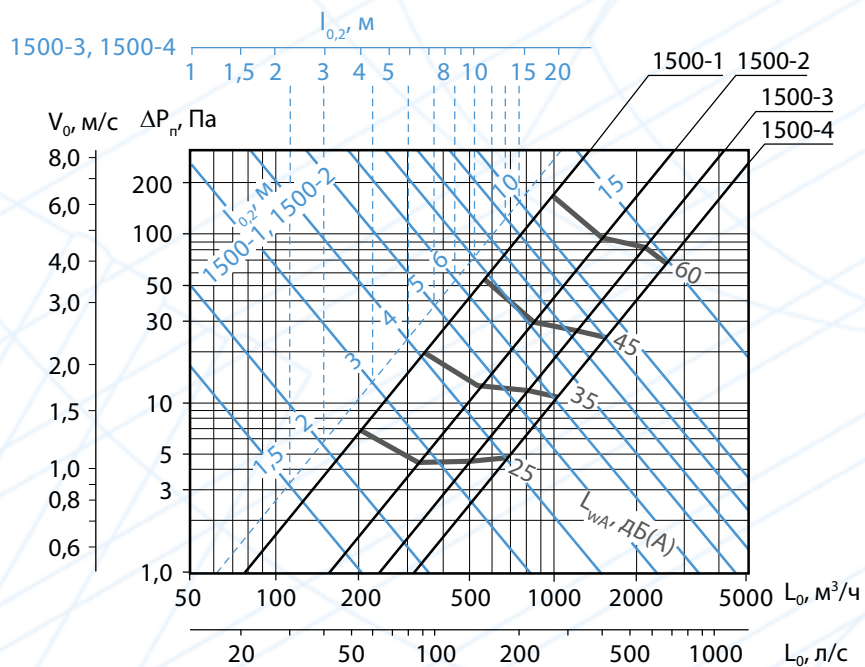
Аэродинамические и акустические характеристики воздухораспределителей КВТ длиной 1500 мм при подаче воздуха в помещение по схеме 4 потоком, направленным в две стороны в плоскости панели
