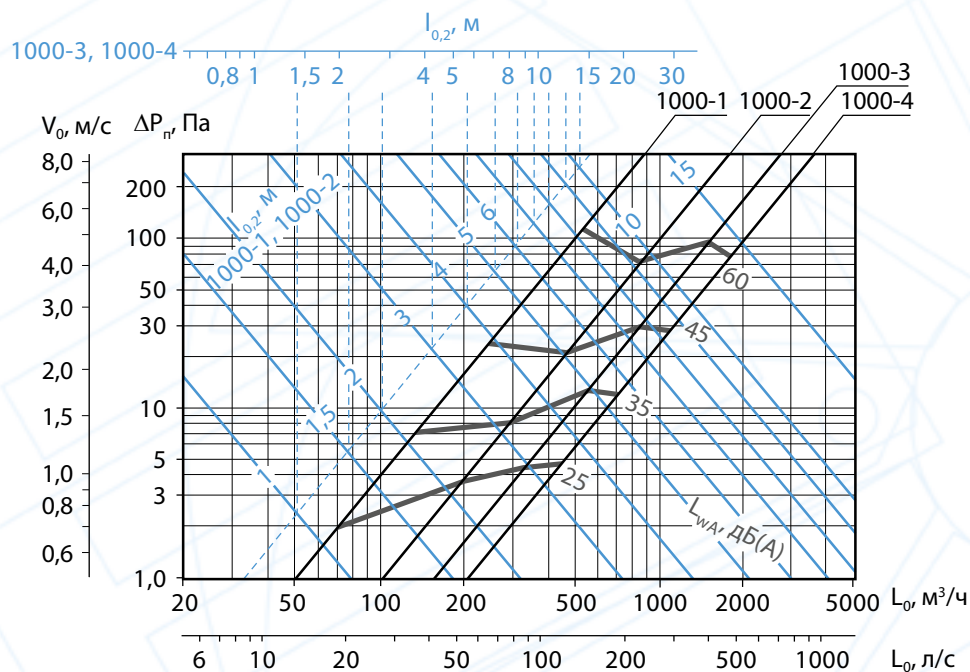
Аэродинамические и акустические характеристики воздухораспределителей КВТ длиной 1000 мм при подаче воздуха в помещение по схеме 4 потоком, направленным в две стороны в плоскости панели
