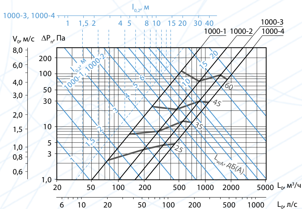
Аэродинамические и акустические характеристики воздухораспределителей КВТ длиной 1000 мм при подаче воздуха в помещение по схеме 3 потоком, направленным в одну сторону в плоскости панели
