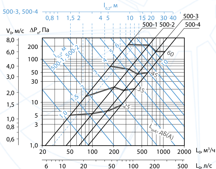
Аэродинамические и акустические характеристики воздухораспределителей КВТ длиной 500 мм при подаче воздуха в помещение по схеме 4 поток, направленным в две стороны в плоскости панели
