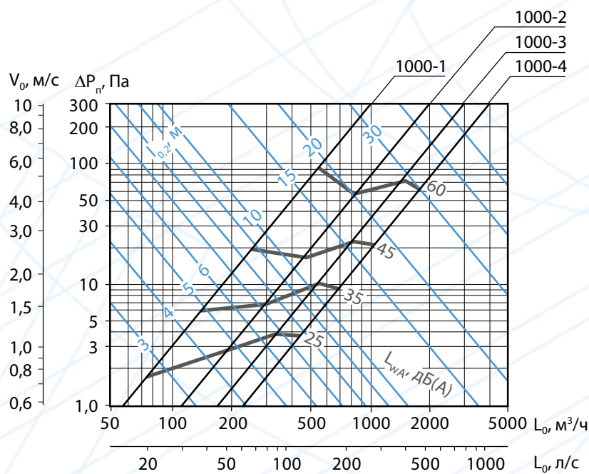
Аэродинамические и акустические характеристики воздухораспределителей ПВТ длиной 1000 мм при подаче воздуха в помещение по схеме 3 потоком, направленным в одну сторону в плоскости панели
