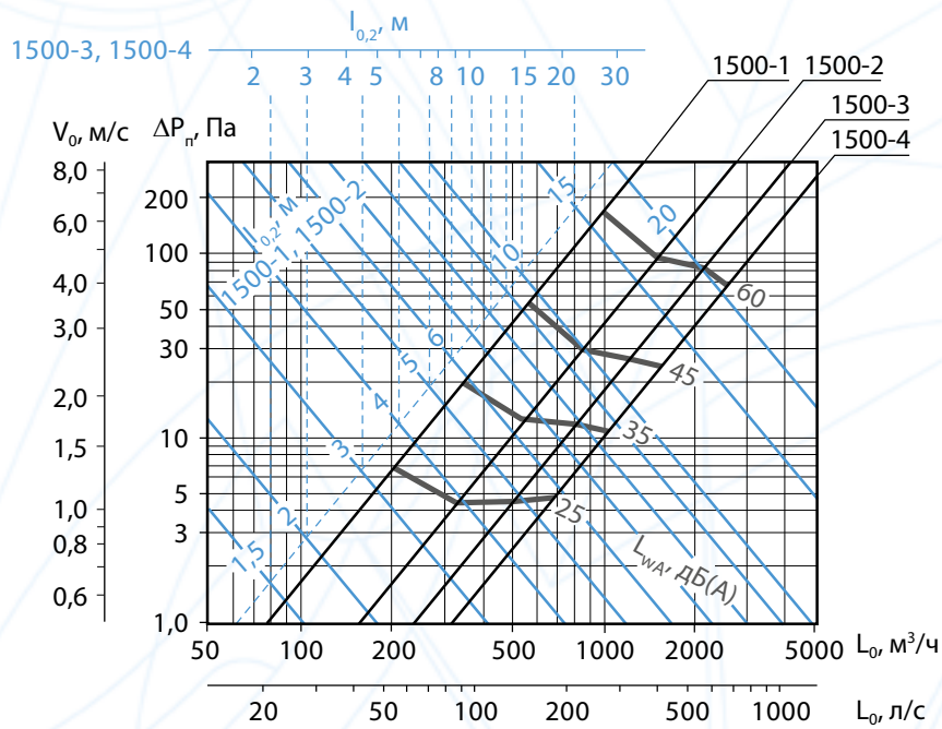
Аэродинамические и акустические характеристики воздухораспределителей КВТ длиной 1500 мм при подаче воздуха в помещение по схеме 3 поток, направленным в одну сторону в плоскости панели
