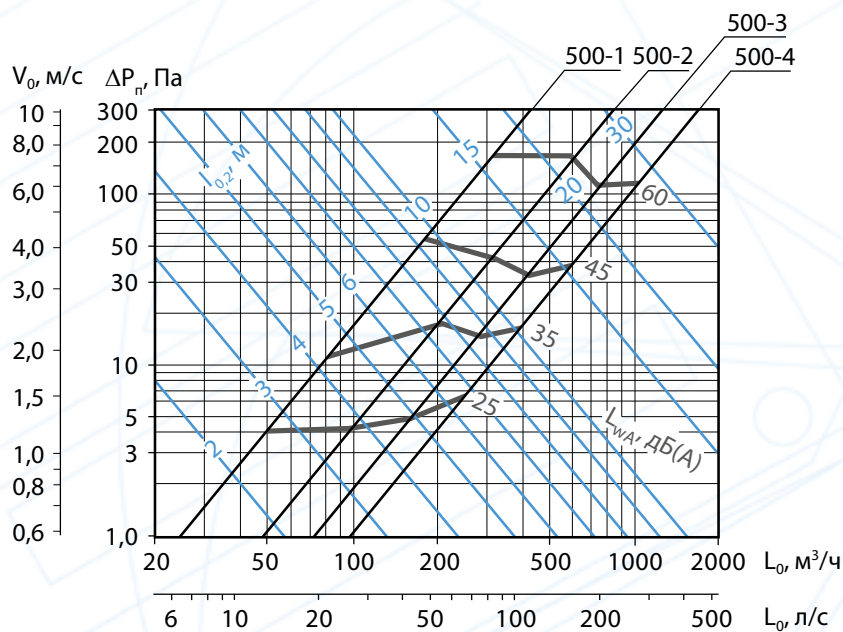
Аэродинамические и акустические характеристики воздухораспределителей ПВТ длиной 500 мм при подаче воздуха в помещение по схеме 3 потоком, направленным в одну сторону в плоскости панели
