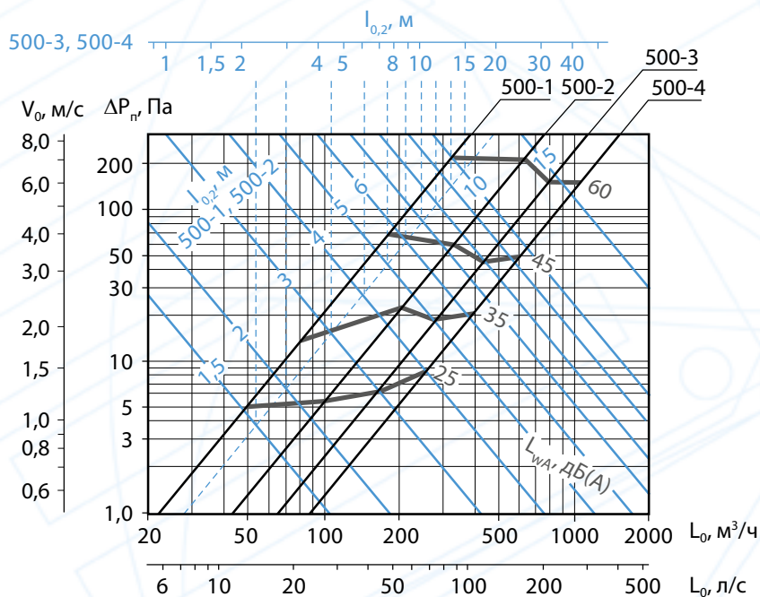
Аэродинамические и акустические характеристики воздухораспределителей КВТ длиной 500 мм при подаче воздуха в помещение по схеме 3 потоком, направленным в одну сторону в плоскости панели
